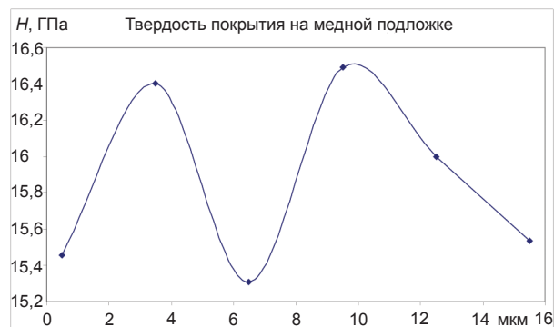
Рис. 7. Нанотвердость покрытия на медной подложке
