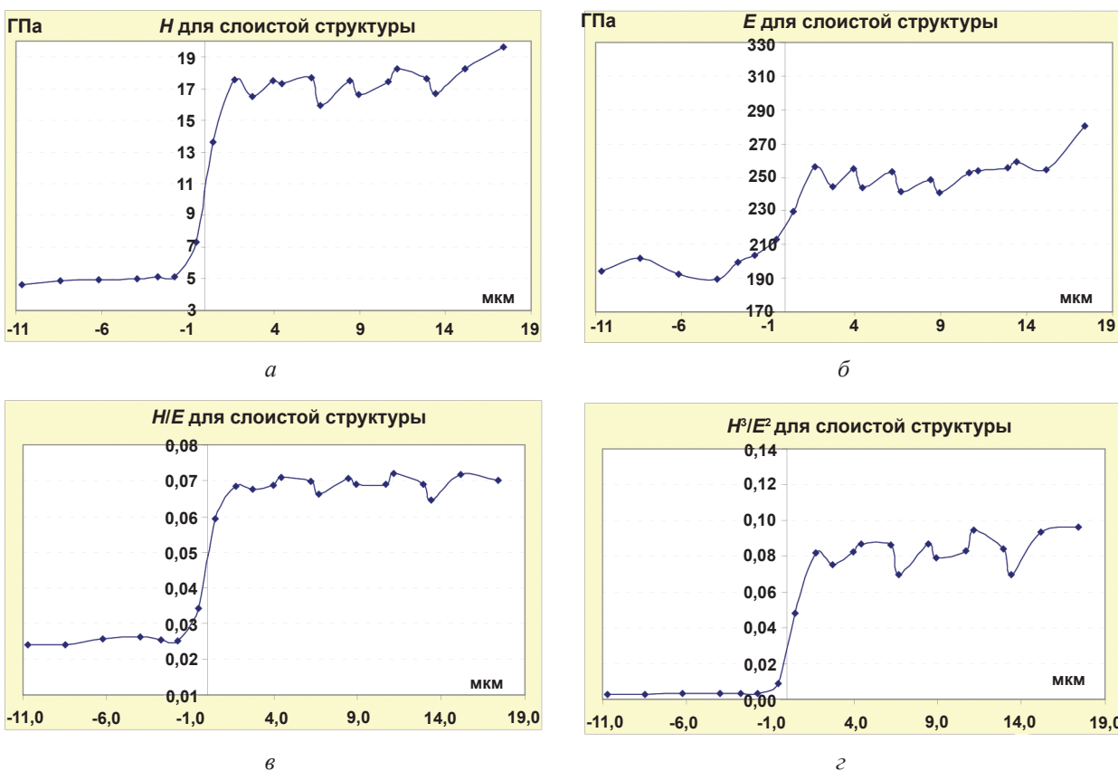
Рис. 3. Физико-механические свойства подложки и покрытия с горизонтально-слоистой структурой
