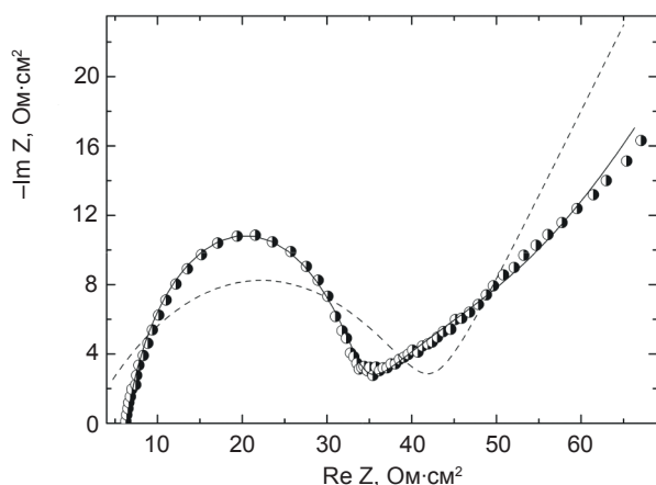
Рис. 5. Графіки Найквіста для системи Li/LiBF 4 + γ-БЛ/InSe. Символи — експериментальний спектр, лінії — спектри, розраховані на основі моделей з рис. 4: a — пунктирна, b — суцільна лінії
