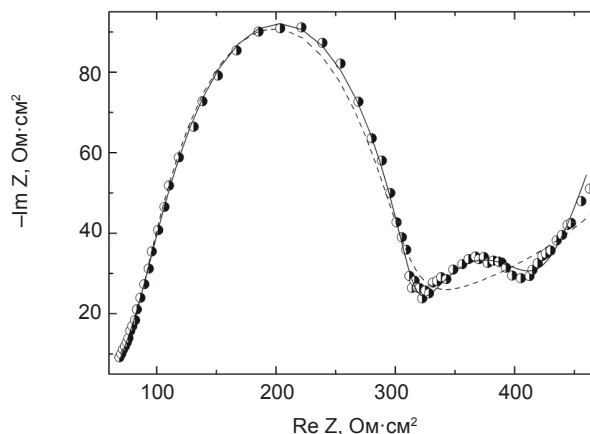
Рис. 6. Графіки Найквіста для системи Li/LiBF 4 + γ-БЛ/Li 0.8 InSe. Символи — експериментальний спектр, лінії — спектри, розраховані на основі моделей з рис. 4: b — пунктирна, v — суцільна лінії
