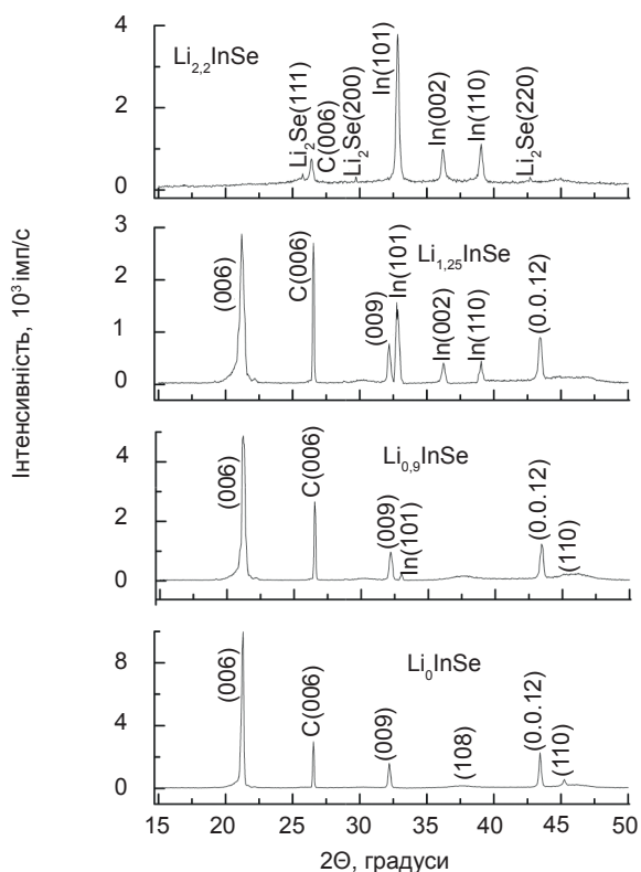
Рис. 2. X -променеві дифрактограми, отримані для системи \text{Li}/\text{LiBF}_4 + \gamma\text{-БЛ}/\text{Li}_x\text{InSe} на різних стадіях розряду. Відбивання від \text{InSe} позначені індексами Міллера, а від утворених фаз — символом фази та індексами Міллера
