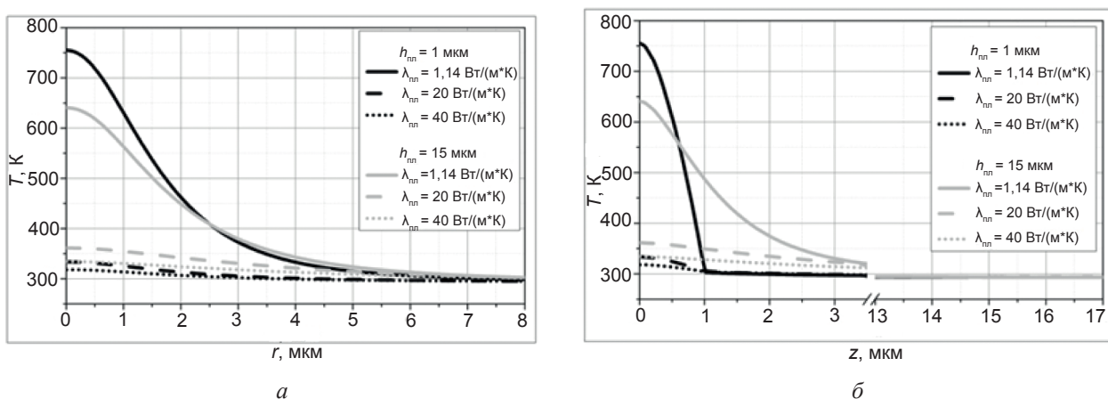
Рис. 8. Влияние теплопроводности пленки на распределение температуры по поверхности (а) и по глубине объекта (б) ( R_{II} = 10 мкм, \text{tg} \delta_{nn} = 1 , C_{nn} = 859 Дж/(кг·К), \tau = 10 мкс, \epsilon_{nn} = 5,3 )
