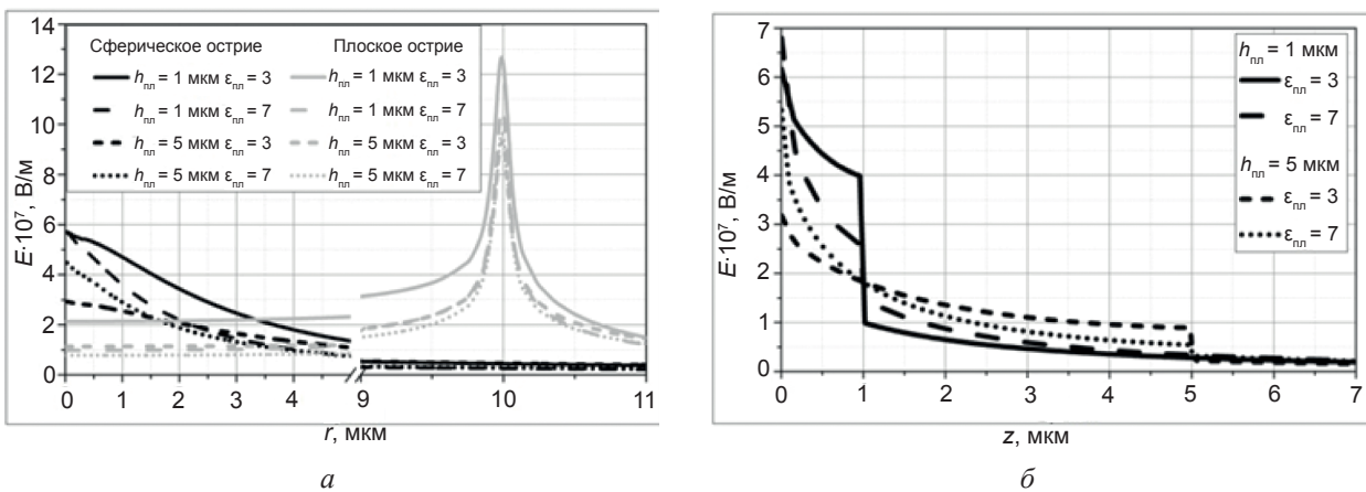
Рис. 4. Распределение СВЧ электрического поля вдоль радиуса острия микромодификатора (а) и по глубине образца (б) ( R_{\text{ш}} = 10 \text{ мкм} , \text{tg} \delta_{\text{пл}} = 0,1 , \tau = 10 \text{ мкс} )
