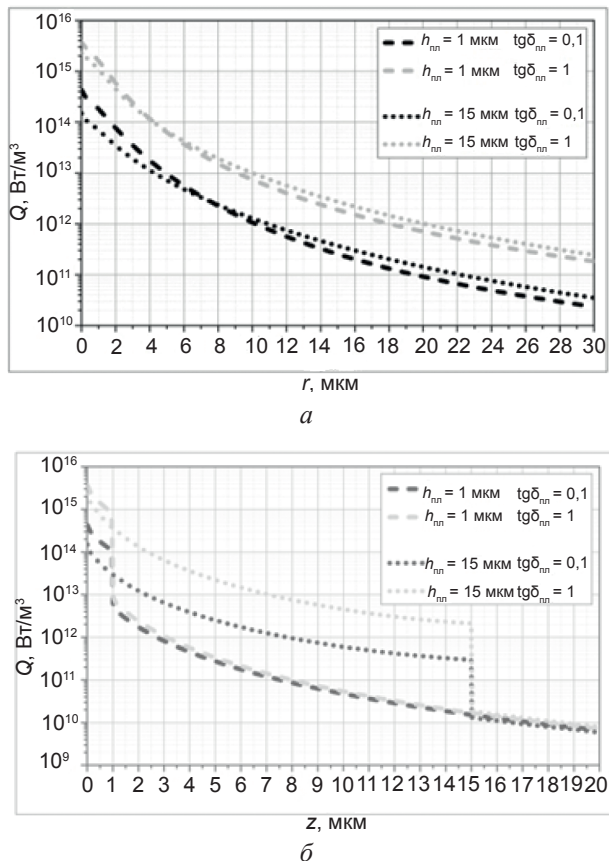
Рис. 5. Влияние толщины пленки и tg\delta_{пл} на распределение тепловыделения по поверхности объекта (а) и по его глубине (б) ( R_{lt} = 10 мкм, \lambda_{пл} = 1,14 Вт/(м·К), C_{подл} = 859 Дж/(кг·К), \tau = 10 мкс)
