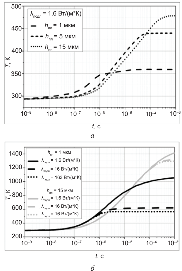
Рис. 6. Кинетика установления пространственного распределения температуры ( R_{lt} = 10 мкм, P = 10 Вт; C_{подл} = 859 Дж/(кг·К), tg\delta_{пл} = 0,1 )
