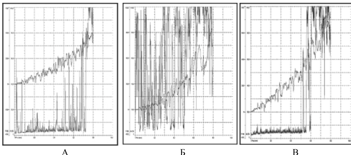
Рис. 7. Спектры акустической эмиссии от образцов с покрытиями: А – активированное, Б – вакуумное, В – активированное (в две стадии).
