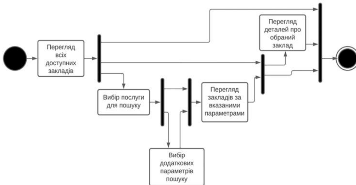
Рис.1 Діаграма активності
