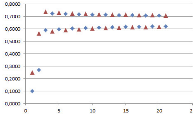
Рис.4. Притягувальний цикл періоду 2 \alpha = 1 + \sqrt{6} ; u_0 = 0,1 ; u_0 = 0,25
