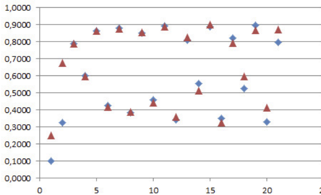
Рис.5. Осциляційні режими довільного періоду \alpha = 3,6 ; u_0 = 0,1 ; u_0 = 0,25
