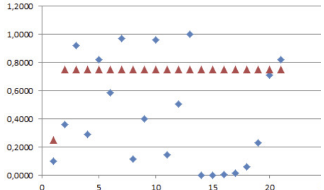
Рис.6. Динамічний хаос \alpha = 4 ; u_0 = 0,1 ; u_0 = 0,25
