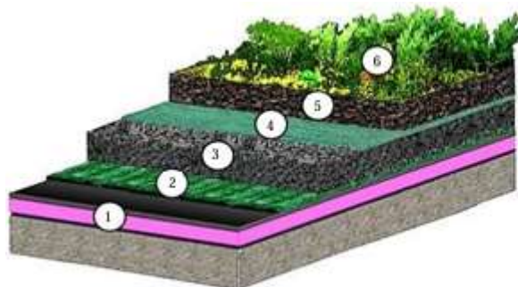
Рис. 2 – Конструктивні рішення зеленого даху [17]
