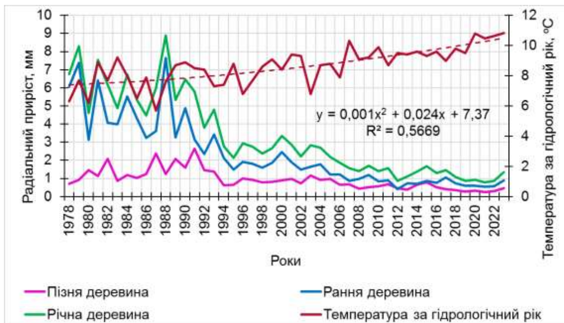
Рис. 1 – Динаміка ранньої, пізньої та однорічної деревини сосни звичайної в насадженні дендропарку Державного Біотехнологічного університету та температура гідрологічного року за даними Харківської метеостанції (N 50°00'47" E 36°13'59")
