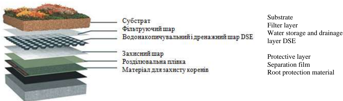
Рис. 1 – Конструктивна структура зеленого даху [17]
