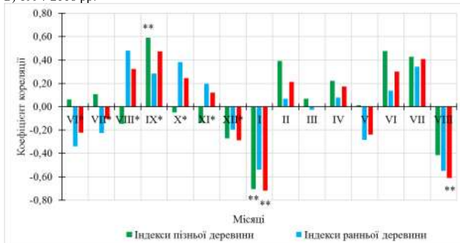
Рис. 3 – Кореляційний аналіз між деревно-кільцевими хронологіями ранньої, пізньої та річної деревини і опадами. Примітка: * – місяці попереднього року; ** – значущість на рівні 0,05
