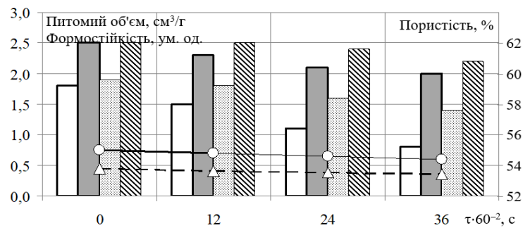
Рис. 5. Питомий об'єм, формостійкість та пористість дослідних зразків житньо-пшеничного хліба в процесі зберігання: – питомий об'єм зразку 1–контролю, – питомий об'єм зразку 3 – з 0,15% СНД, – пористість зразку 1–контролю, – пористість зразку 3 – з 0,15% СНД, – формостійкість зразку 1–контролю, – формостійкість зразку 3 – з 0,15% СНД
