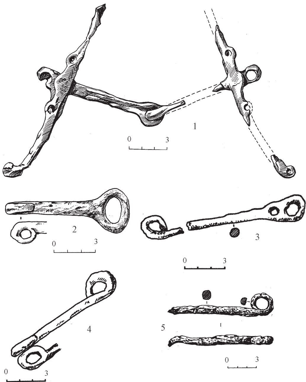
Рис. 7. Железные удила раннескифского времени Северного Кавказа:
