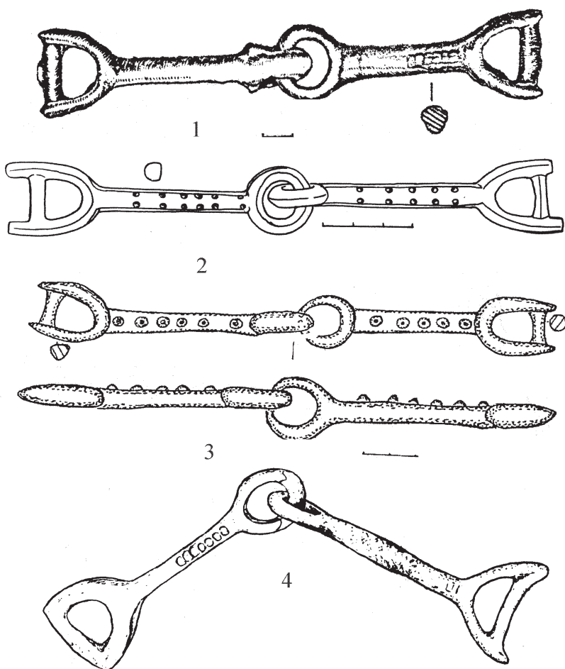
Рис. 3. Бронзовые стремяковидные удила с орнаментированными грызлами лесостепной Украины: 1 – Яснозорье, курган 6; 2 – погребение 2 Репяховатой Могила; 3 – Гуляй-Город, курган 38; 4 – Старшая Могила
