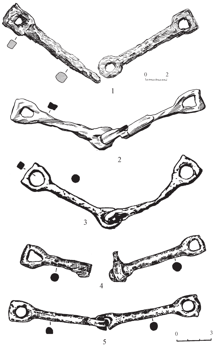
Рис. 4. Железные стремячквидные удила Северного Кавказа:
