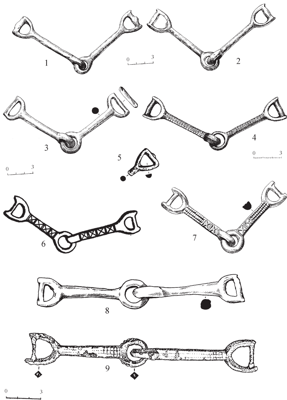
Рис. 1. Бронзовые стремячковые удила Северного Кавказа:
