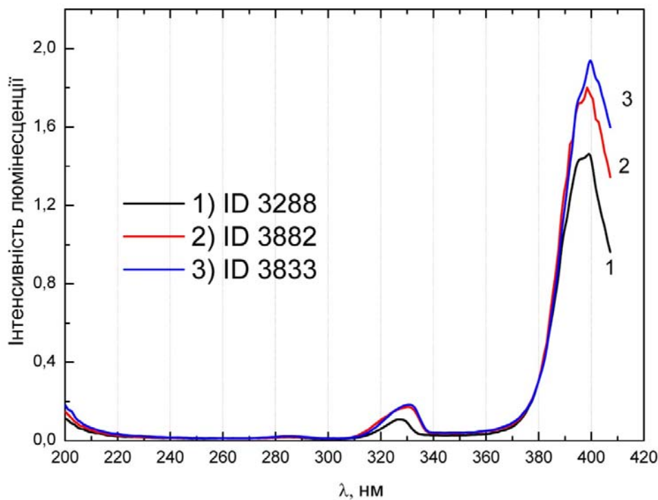
Рис. 5. Спектри збудження люмінесценції порошкових зразків ID 3288 (крива 1), ID 3882 (крива 2) та ID 3833 (крива 3) для довжини випромінювання \lambda_{\text{люм}}=455 нм. В спектрі можна виділити дві широкі смуги з максимумами при 330 та 400 нм.
