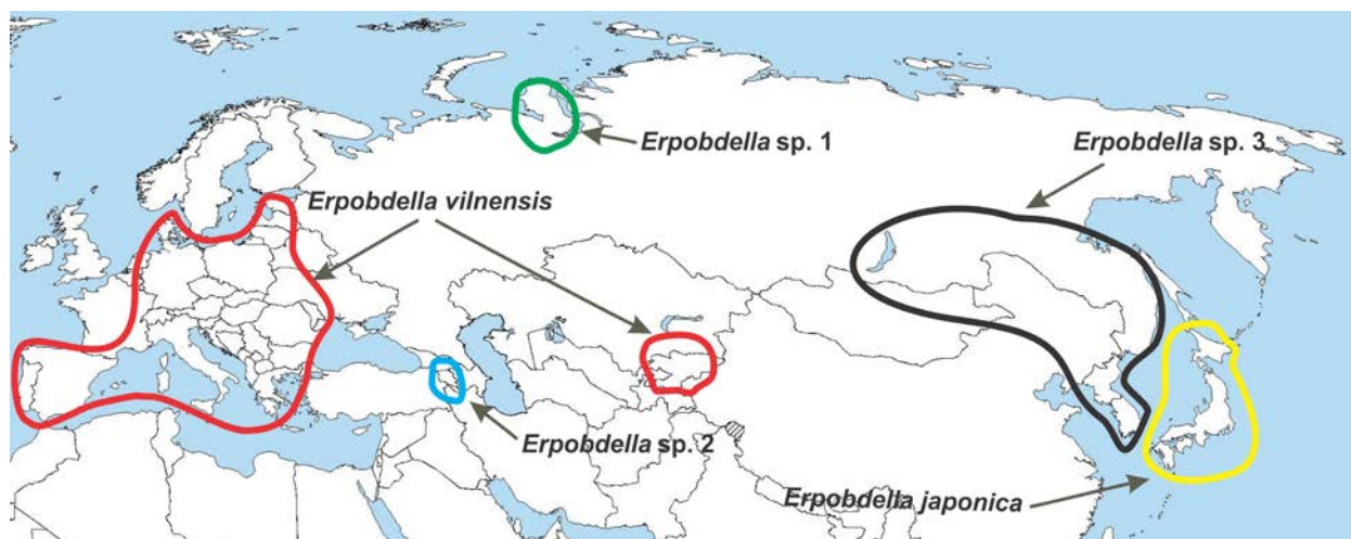
Рис. 2. Ареали споріднених видів глоткових п'явок, що не мають наземних стадій у своєму життєвому циклі, розподілені в напрямку із заходу на схід. Їхнє походження зумовлено виникненням географічних бар'єрів у минулому і географічною ізоляцією
