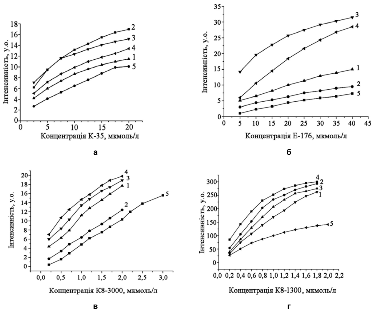
Рис. 5. Інтенсивність флуоресценції зондів К-35 (а), E-176 (б), K8-3000 (в) і K8-1300 (г) в ЕШНП (1), в ЕСС (2), в ЕСЦС (3), в ЕСЦП (4), в буфері (5)
