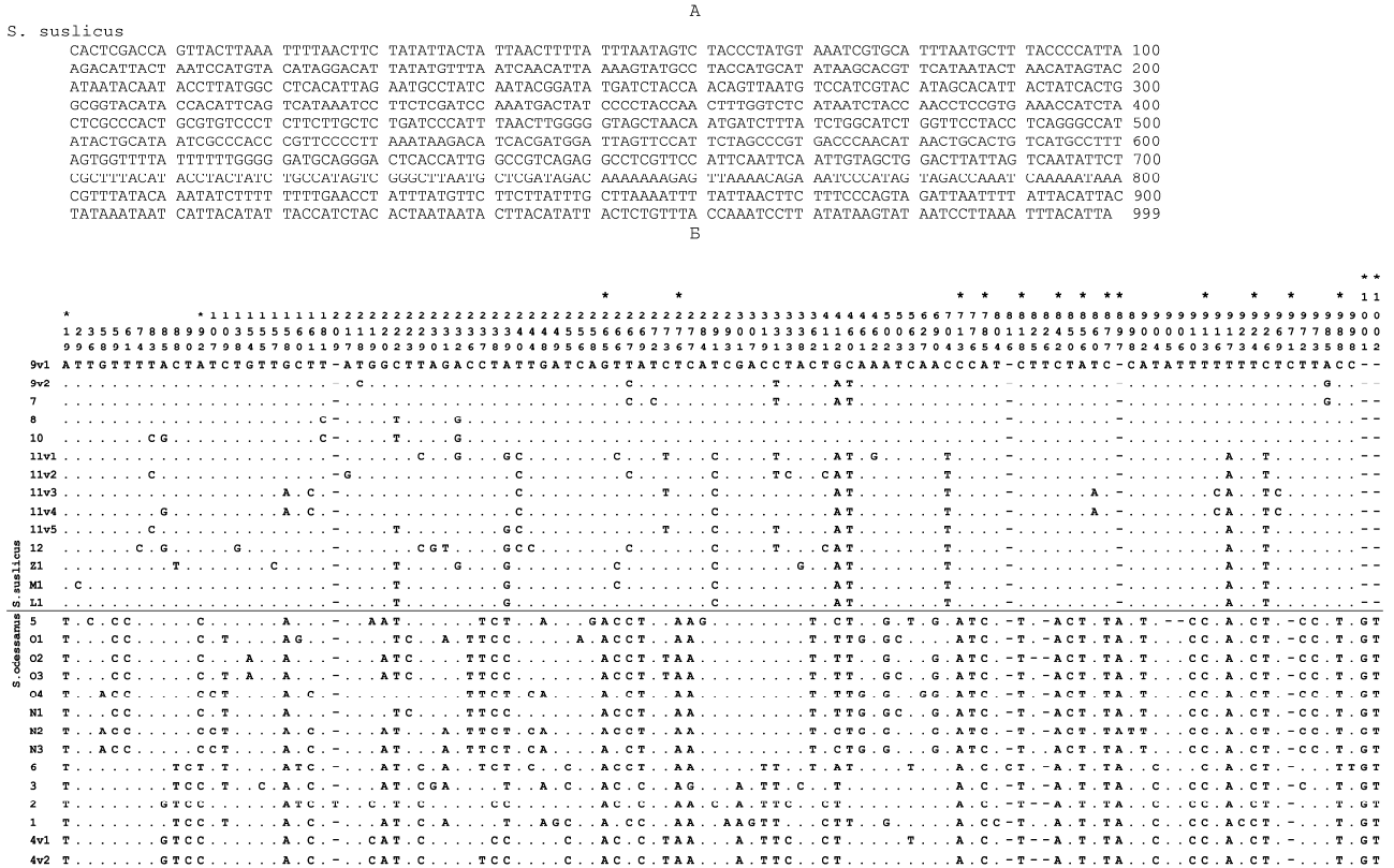
Рис. 2. А – первичная структура контрольного региона мтДНК S. suslicus (популяция 9, гаплотип 9v1); Б – варианты контрольного региона мтДНК крапчатых сусликов. Приведены только вариабельные позиции, нумерация которых соответствует полным структурам, выровненным относительно гаплотипа 9v1. Точками обозначены идентичные нуклеотиды, тире – делеции, звездочками обозначены маркерные замены, отличающие 34- и 36-хромосомные формы. Слева обозначения гаплотипов, включающие обозначение локалитета в соответствии с рис. 1 и табл. и вариант гаплотипа в локалитете при наличии изменчивости
